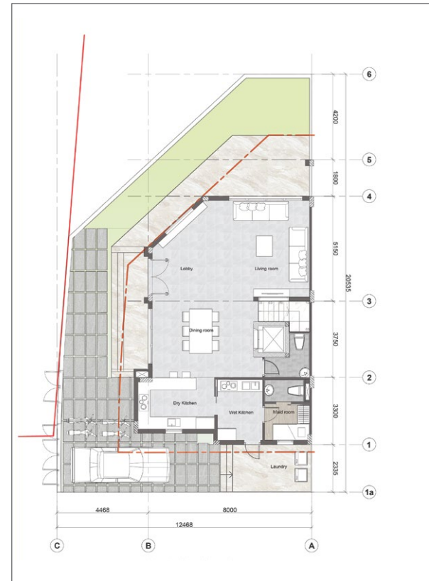
1 1 ST FLOOR PLAN MẶT BẰNG TẦNG 1
